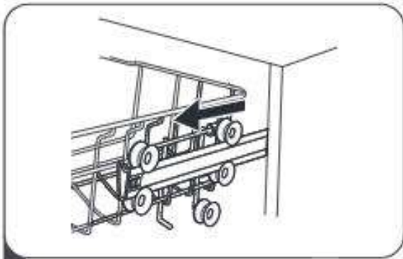
1 Τραβήξτε το πάνω καλάθι.
