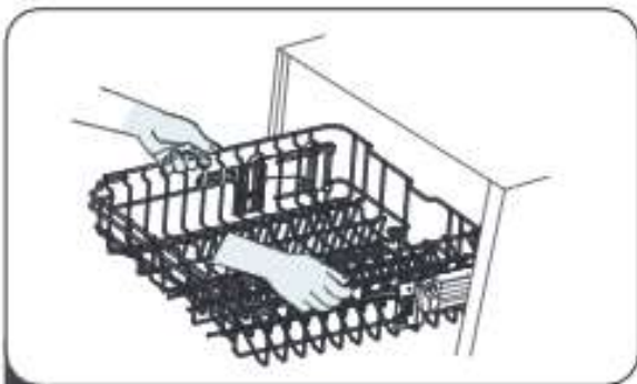
1 Για να σηκώσετε το άνω καλάθι απλώς ανυψώστε το καλάθι στο κέντρο κάθε πλευράς έως ότου το καλάθι ασφαλίσει στην άνω θέση. Δεν είναι απαραίτητο να σηκώσετε τη λαβή ρύθμισης.
