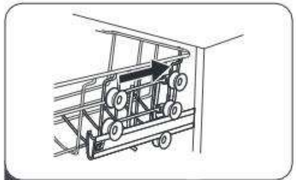
4 Σπρώξτε μέσα το πάνω καλάθι.
