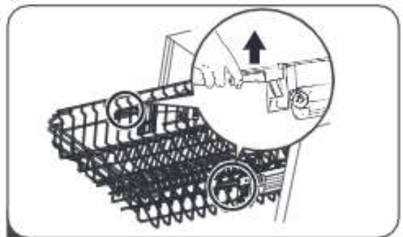
2 Για να κατεβάσετε το πάνω καλάθι, σηκώστε τις λαβές ρύθμισης σε κάθε πλευρά για να απελευθερώσετε το καλάθι και κατεβάστε το στην κάτω θέση.
